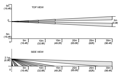
FIG. 6 - LONG RANGE CURTAIN LENS
