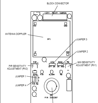
FIG. 4 - PCB LAYOUT
